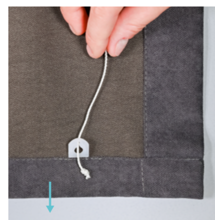
krok 8 | Przelóż sznurek przez oczka i włóż do zaczepu dolnego
